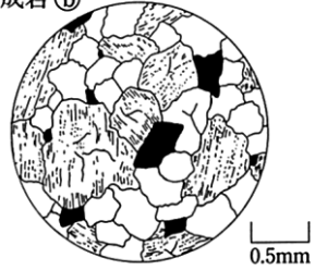
火成岩 ②
