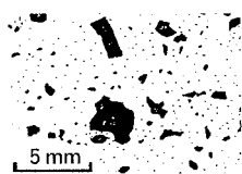
図2 火成岩B
