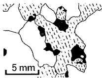
図1 火成岩A
