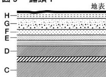
図3 露頭Y
