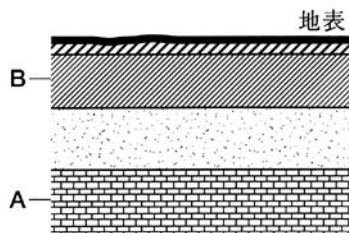
図2 露頭X
