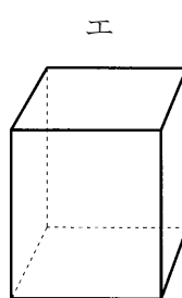
直方体
