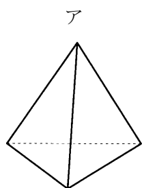
三角すい
