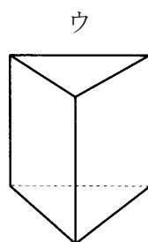
三角柱
