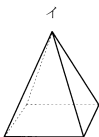
四角すい
